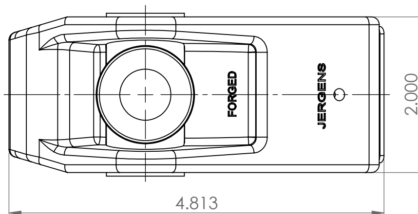
TOP
