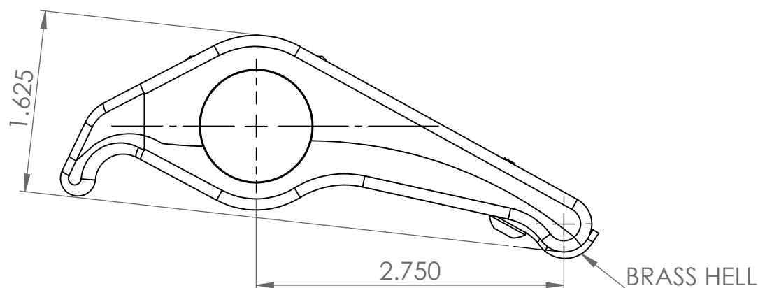
TOP
