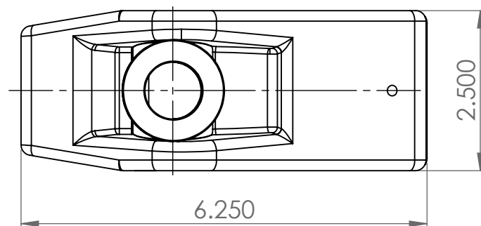
TOP
