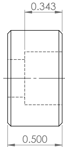
LEFT SIDE
