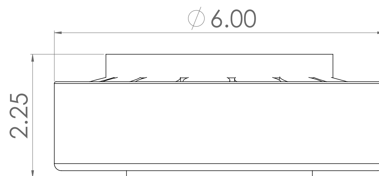
TOP
