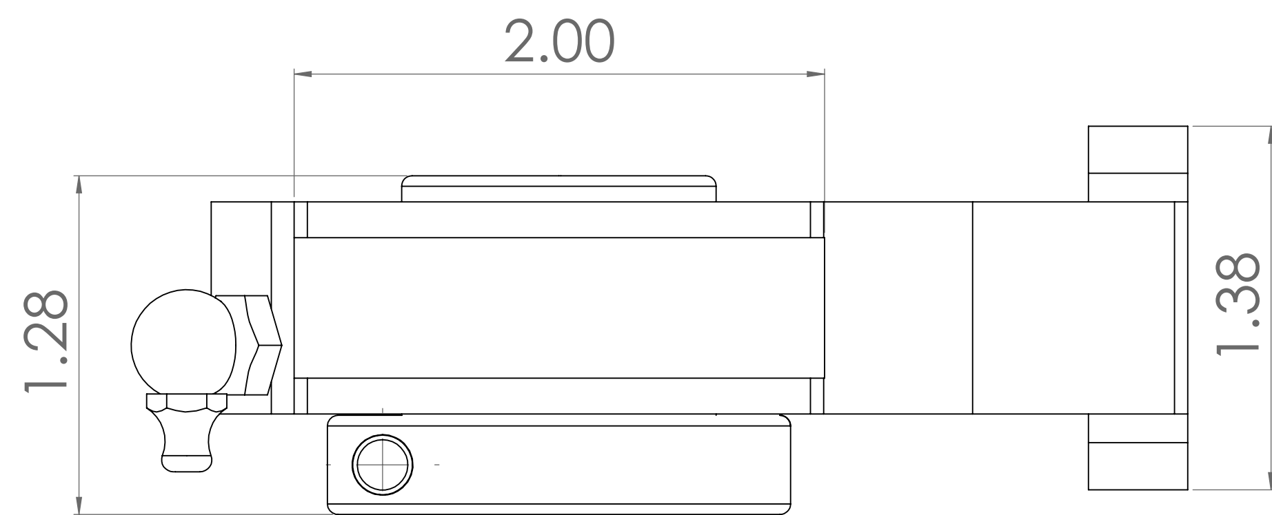
TOP
